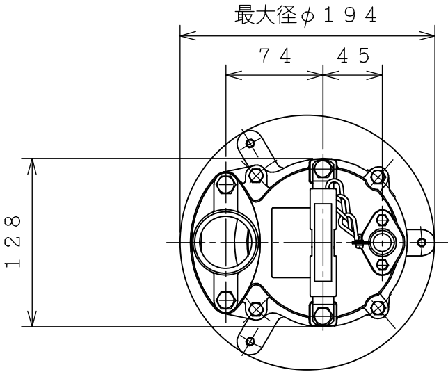
外形寸法図
