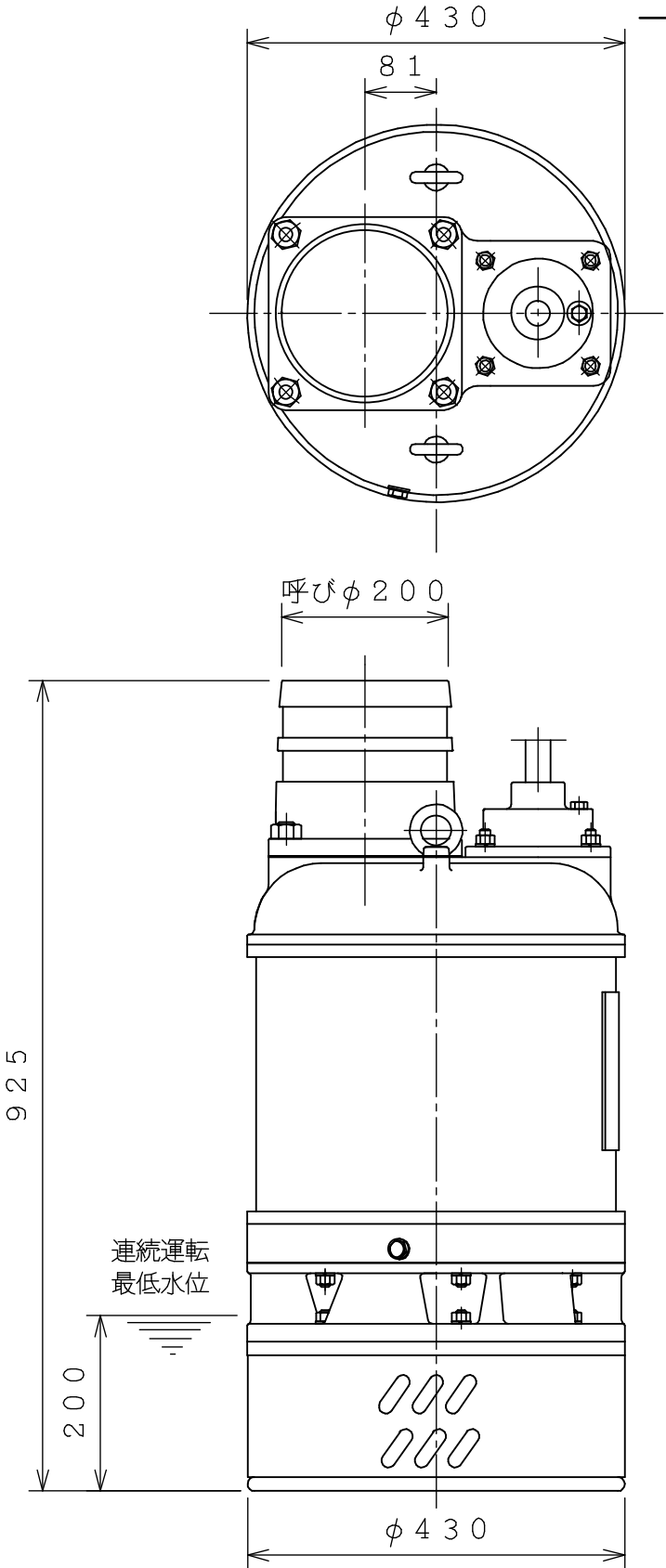
外形寸法図
