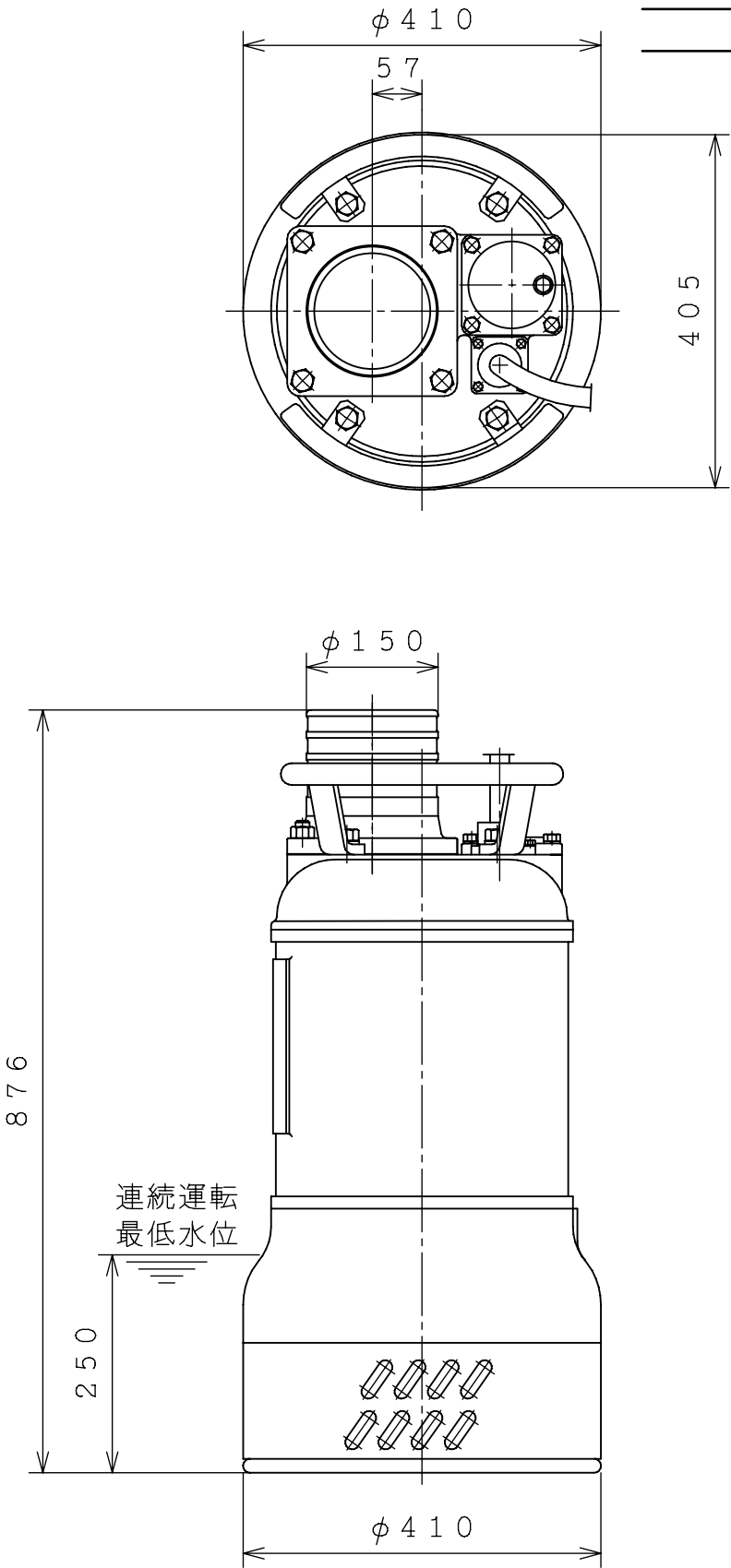
外形寸法図
