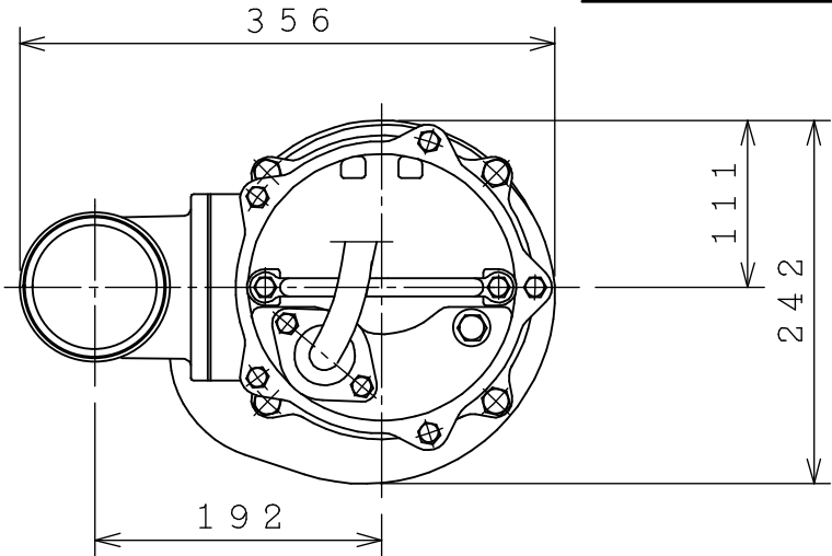
外形寸法図
