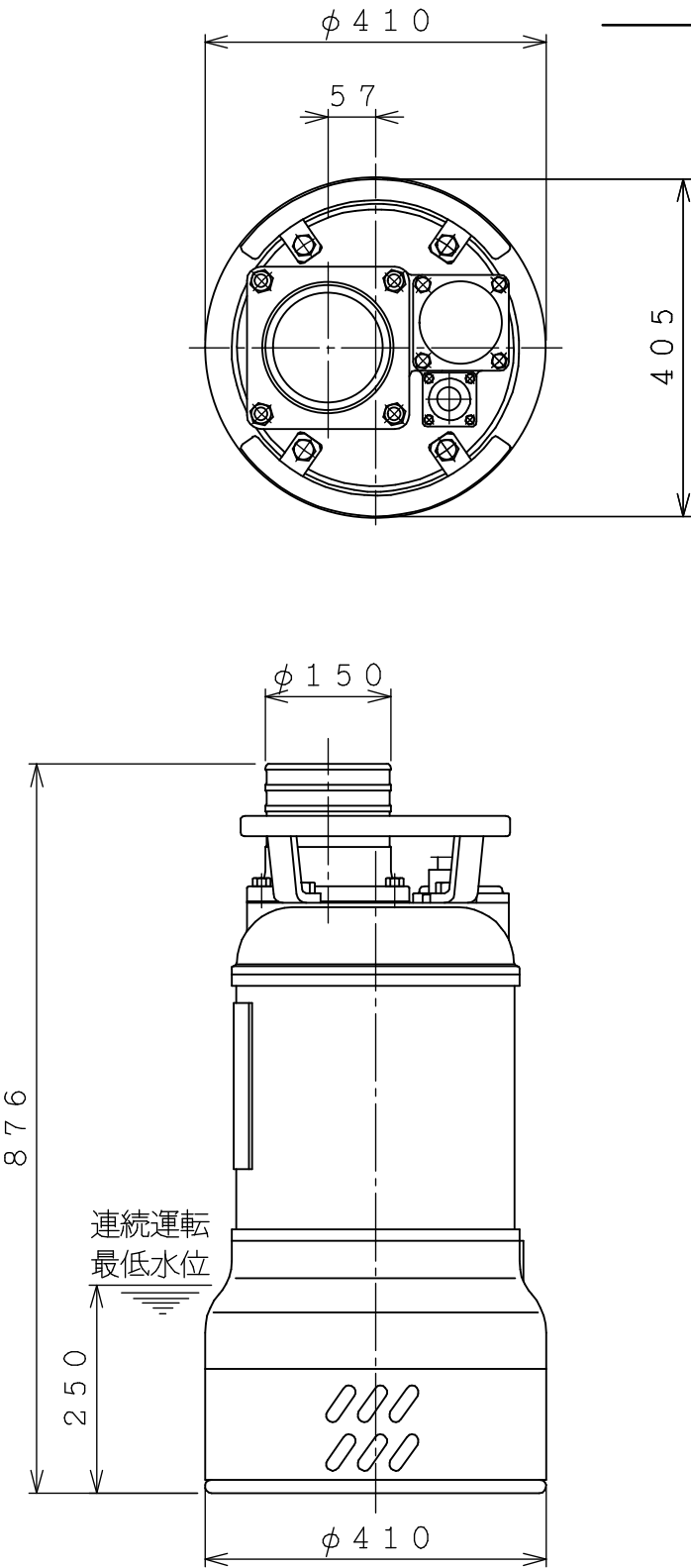
外形寸法図
