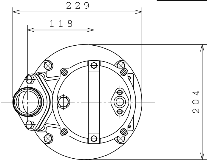
外形寸法図
