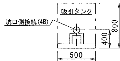
坑口側面図
