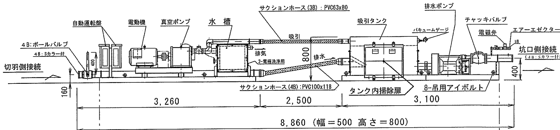
坑口側面図
